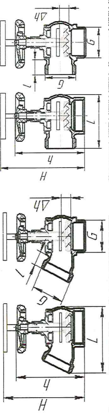
Исполнение 1: КПЛМ, КПЧМ, КПЧМ, КПЧМ Исполнение 2: КПЛМ, КПЧМ, КПЧМ, КПЧМ Рисунок 1—Внешний вид клапанов угловых моделей КПЛ, КПЧ, КПЧ, КПЧ и КПЛМ, КПЧМ, КПЧМ
