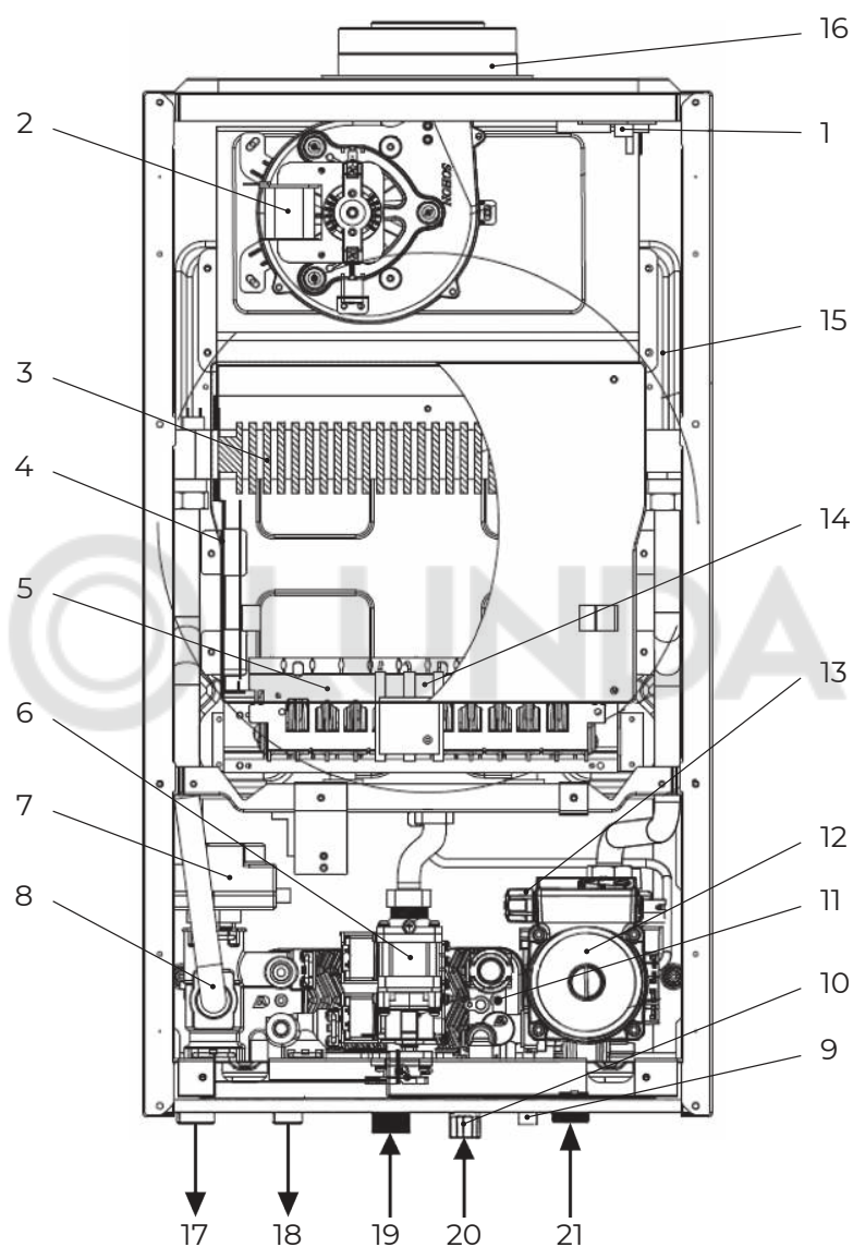
Рис. 3. Общая схема котлов В30 28 С (Wi-Fi), 32 С (Wi-Fi), 36 С (Wi-Fi).
