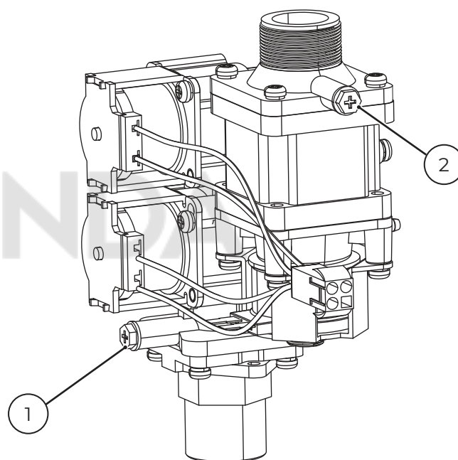
Рис. 40. Газовый клапан.
