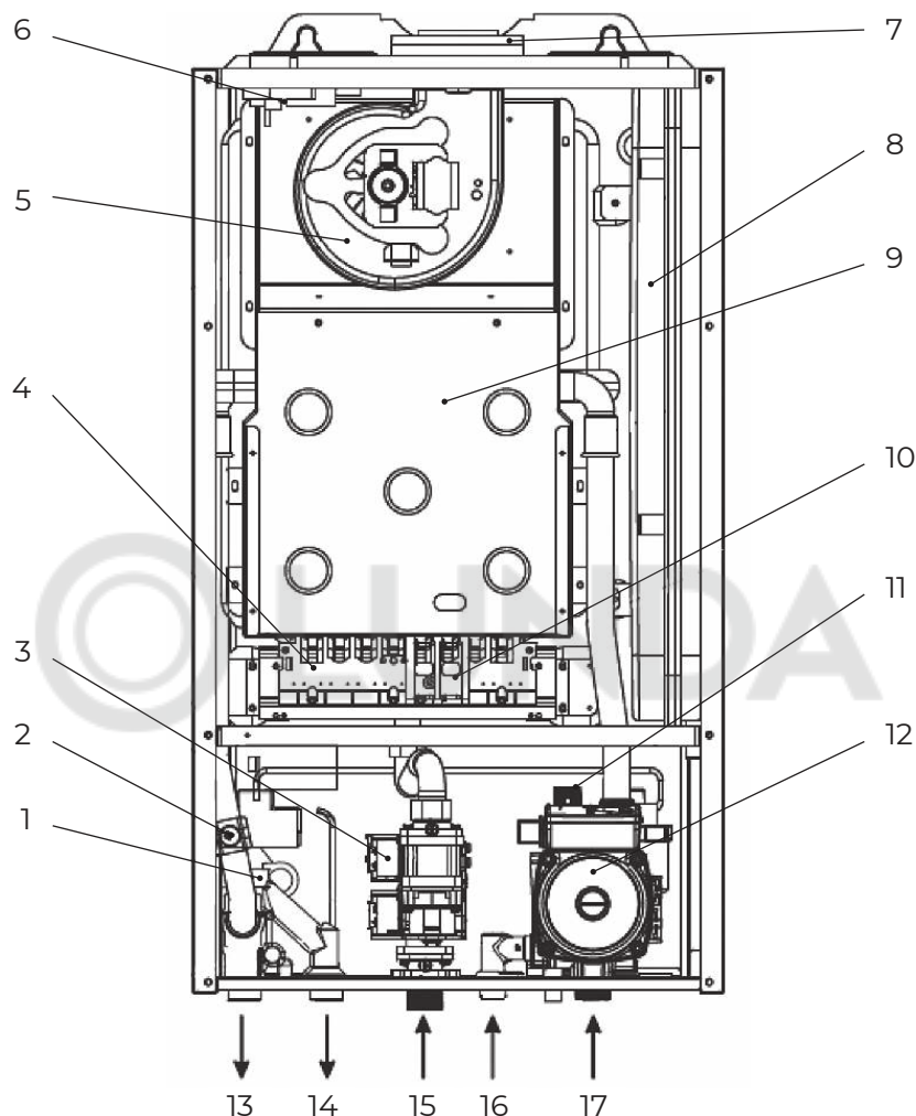
Рис. 4. Общая схема котлов В30 18 Н (Wi-Fi), 24 Н (Wi-Fi).
