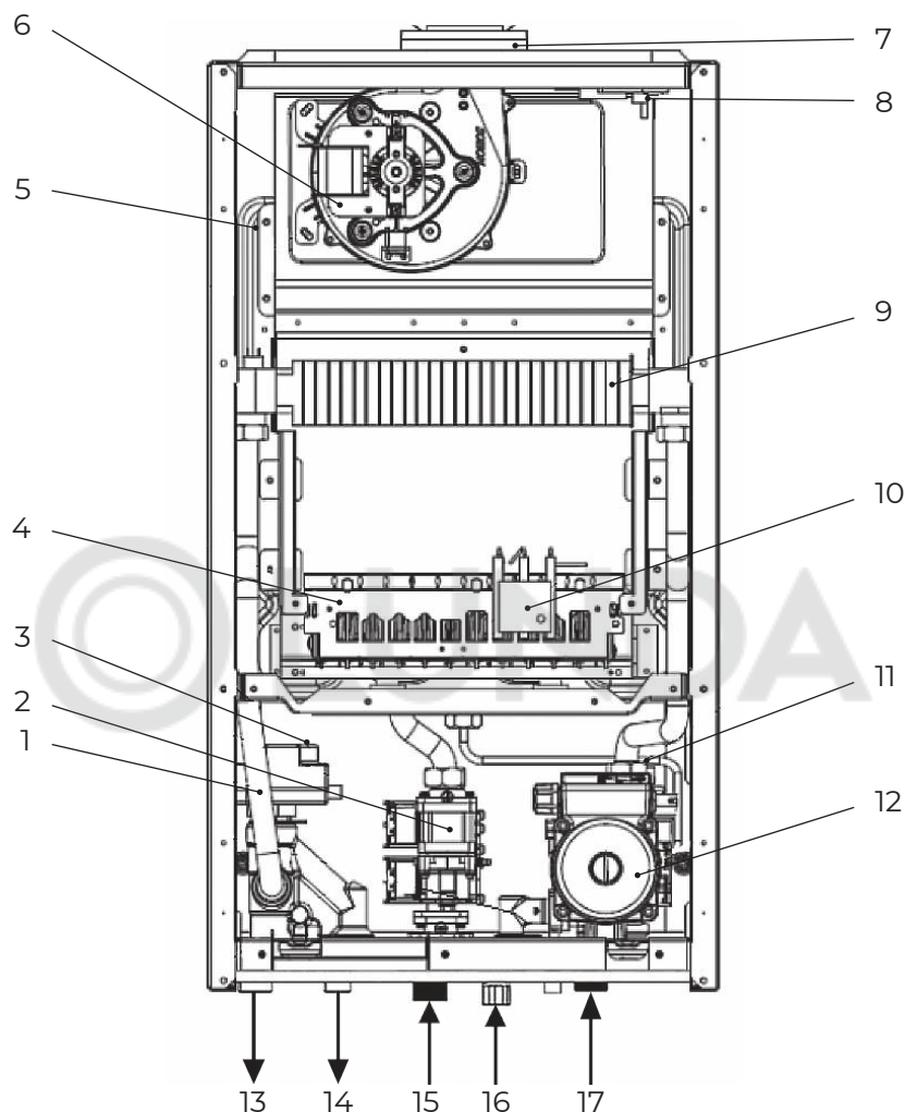
Рис. 5. Общая схема котлов B30 28 H (Wi-Fi), 32 H (Wi-Fi), 36 H (Wi-Fi).
