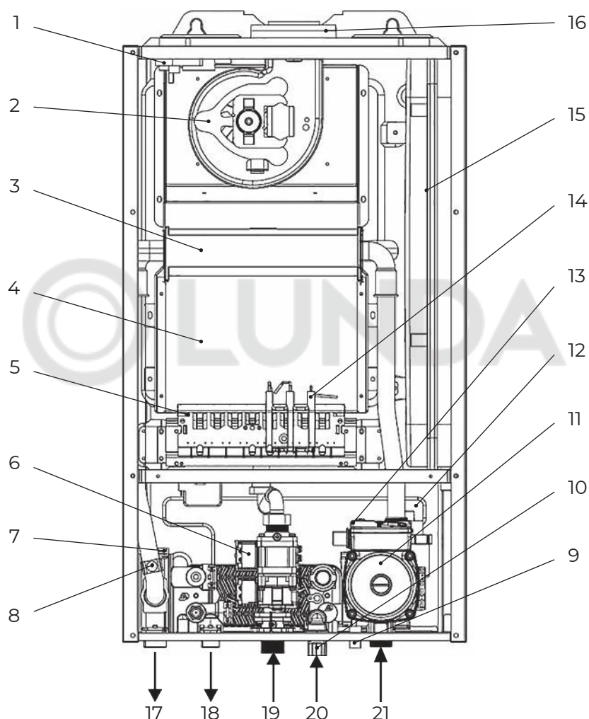
Рис. 2. Общая схема котлов В30 18 С (Wi-Fi), 24 С (Wi-Fi).
