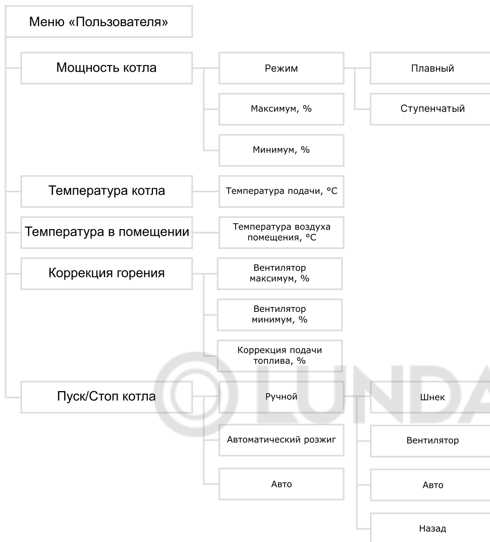
Рис.15 Блок-схема меню пользователя
