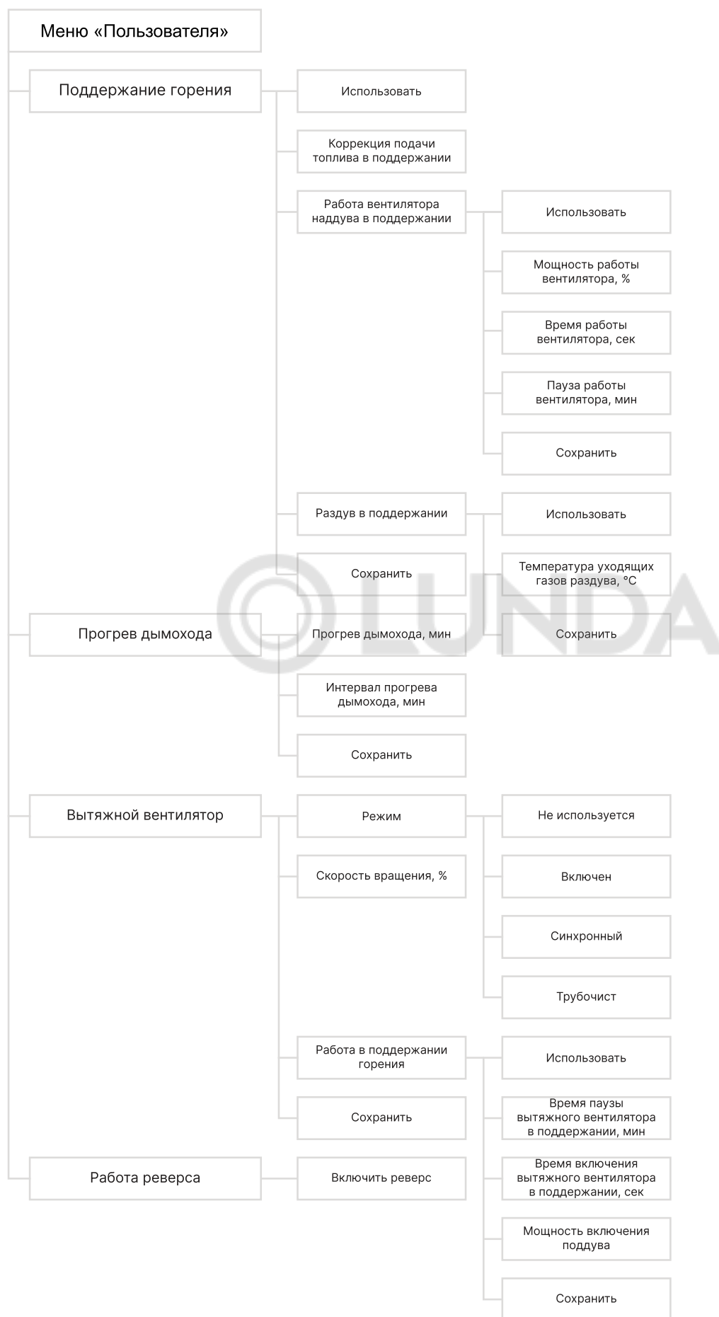
Рис.19 Блок-схема меню пользователя (продолжение)
