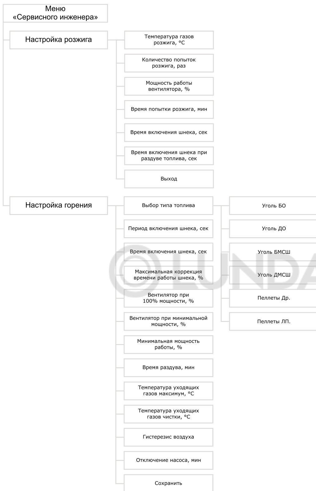
Рис.26 Блок-схема меню сервисного инженера (продолжение)
