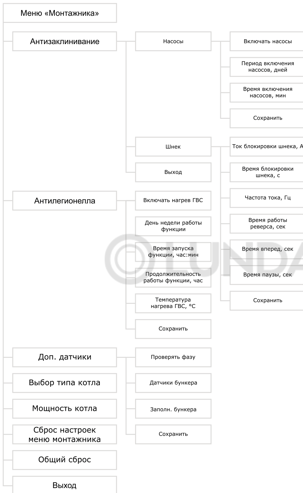
Рис.24 Блок-схема меню монтажника (продолжение)
