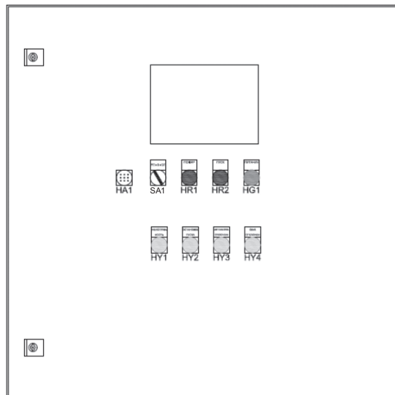
Рис. 11 Прибор управления пожарный Control MX
