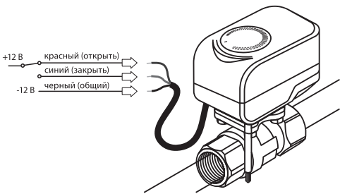
Рис. 2 Электрическая схема подключения крана с электроприводом серии Neptun Standard 12B
