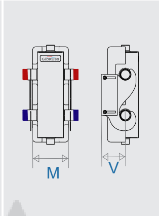
Рис.2. Монтажные размеры гидрострелок в теплоизоляции GR/GRSS-60/80
