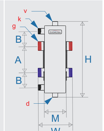
Рис.3. Габариты и подключения резьбовых гидрострелок GR/GRSS-100/150
