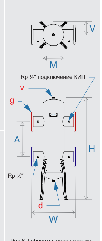
Рис.6. Габариты, подключения и монтажные размеры фланцевых гидрострелок GR/GRSS-600..3000
