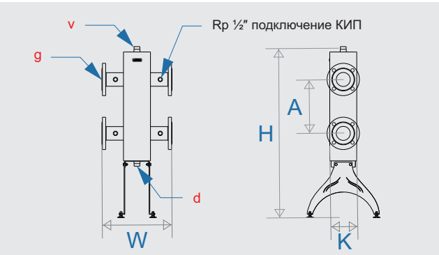
Рис.5. Габариты, подключения и монтажные размеры фланцевых гидравлических разделителей с корпусом квадратного сечения GR/GRSS-400
