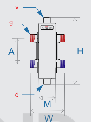
Рис.1. Габариты и подключения резьбовых гидрострелок GR/GRSS-40/60/80/250
