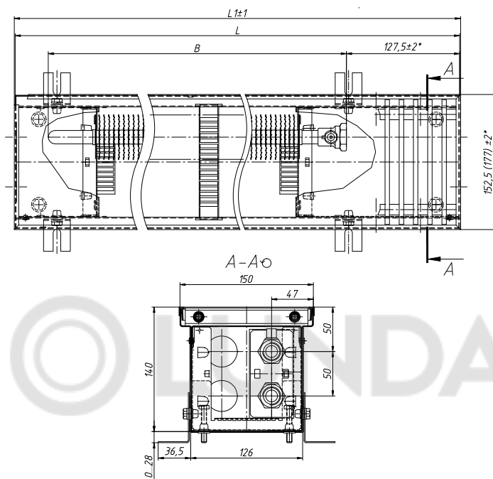
КРК 15.19.060...400
