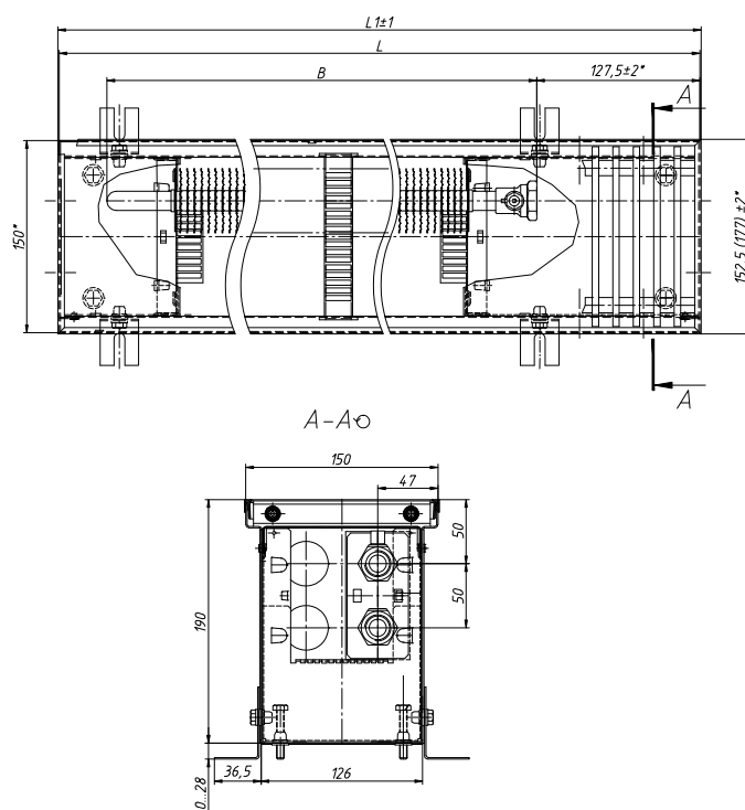
КРК 15.19.060...400
