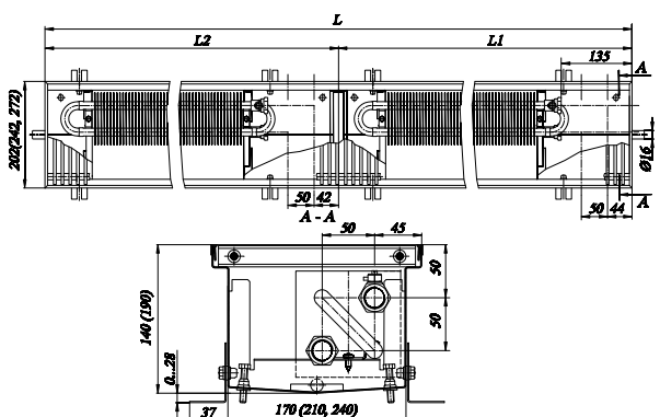
КРОК 20(24, 27).14(19).320...600-ПП
