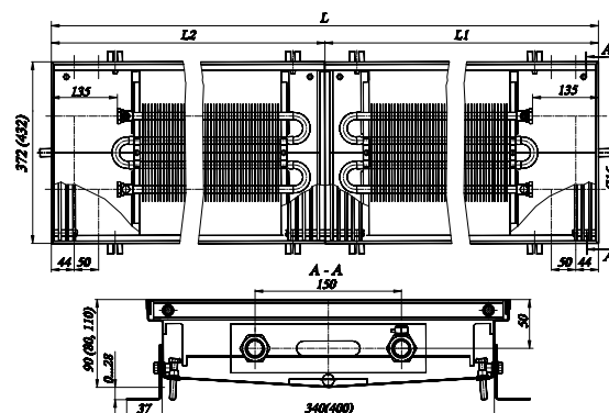
КРОК 37(43).08(09, 11).320...600-ПП
