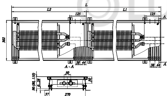
КРК 30.08(09,11).320...600-ПП
