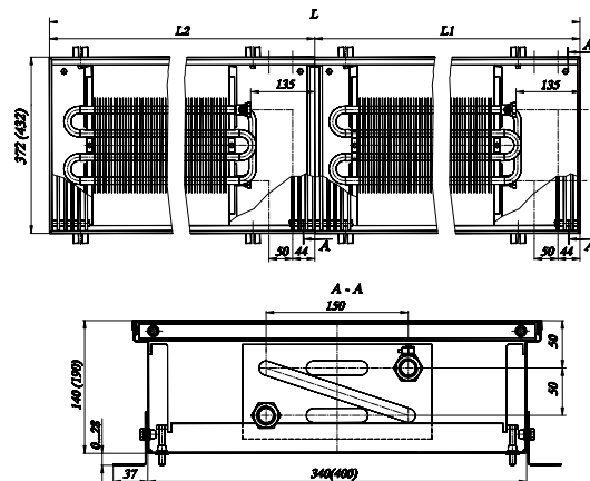
КРК 37(43).14(19).320...600-ПП
