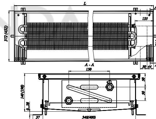
КРОК 37(43).14(19).060...310-П
