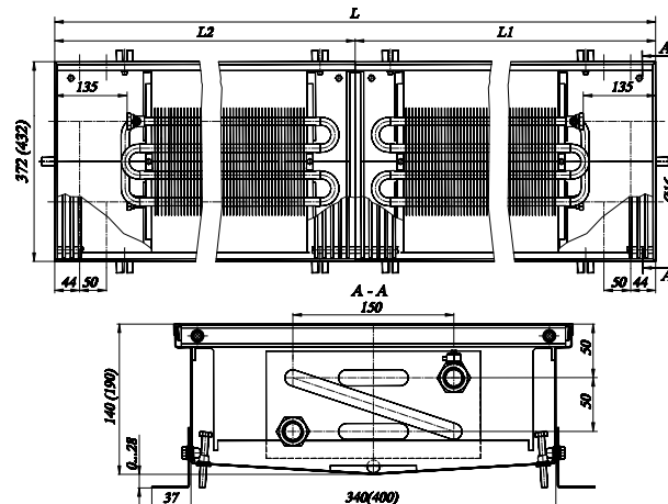
КРОК 37(43).14(19).320...600-ЛП
