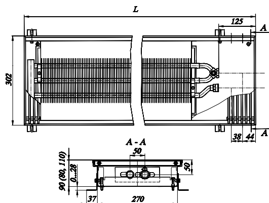
КРК 30.08(09,11).060...310-П
