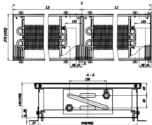
КРК 37(43).14(19).320...600-ПП
