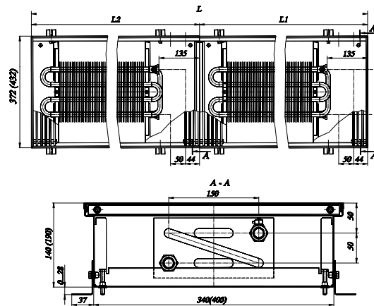
КРК 37(43).14(19).320...600-ПП
