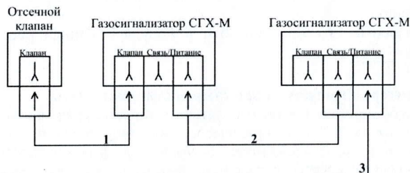
Схема подключения газосигнализаторов СГХ-М(П).
