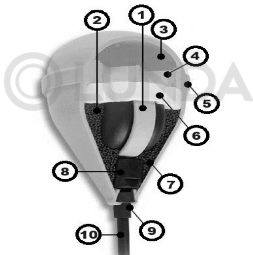
Рис. 1 Конструкция датчика уровня FS-1
