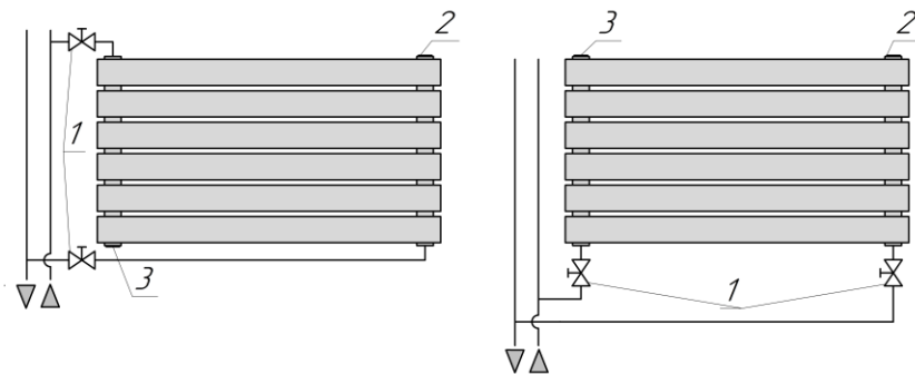
Рис. 3. 1. Вентиль (кран). 2. Кран Маевского-воздухоотводчик. 3. Пробка глухая.
