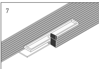
7 Нанесите клеевой слой по периметру желоба
