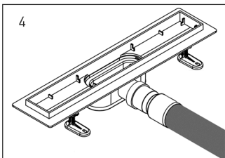
4 Установите желоб, присоедините сифон к канализации
