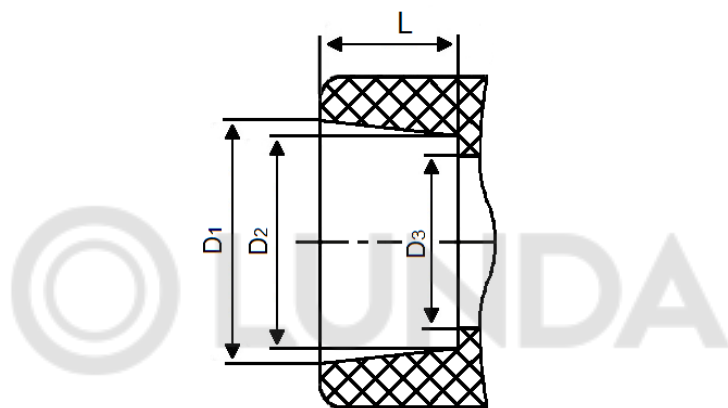
Рис 2. Раструбная часть фитингов серии PRO
