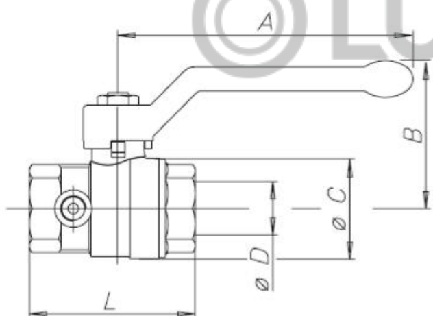
Рис. 5. Габаритные и присоединительные размеры
