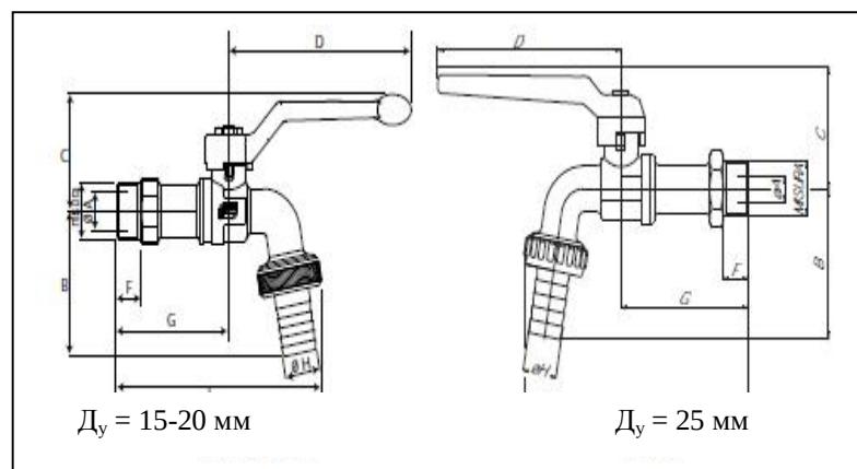
Рис.12. Габаритные размеры
