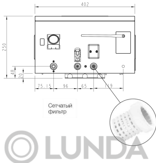
Рис. 19. Сетчатый фильтр
