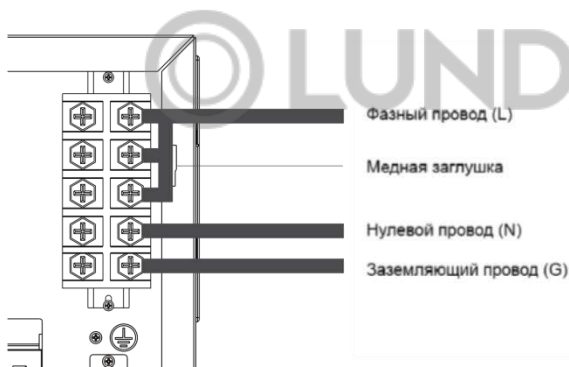
Рис. 10. Однофазное подключение прибора
