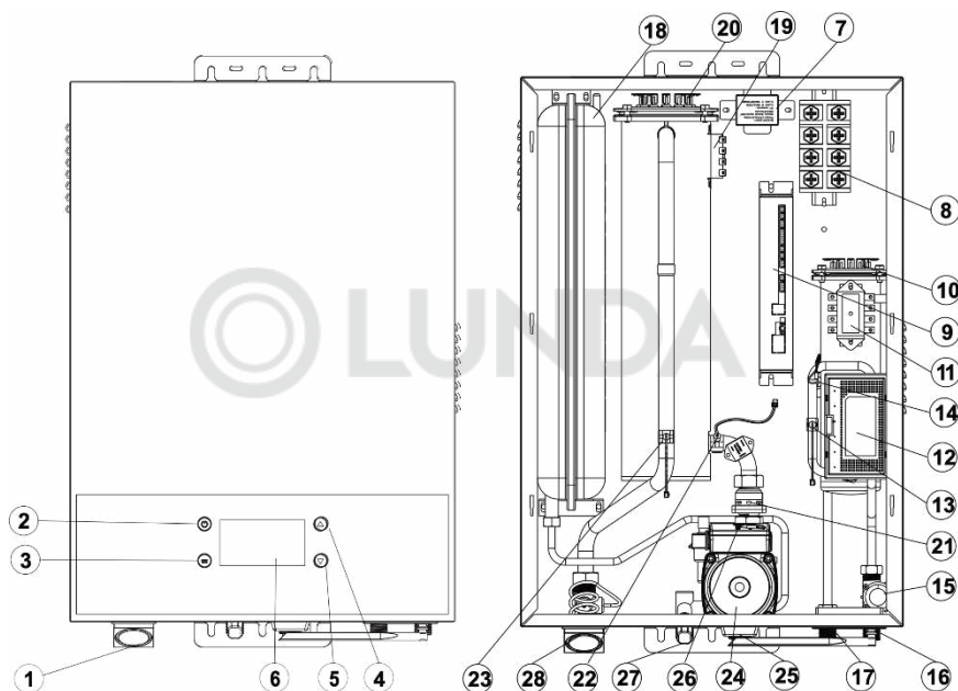
Рис. 1. Конструкция изделия
