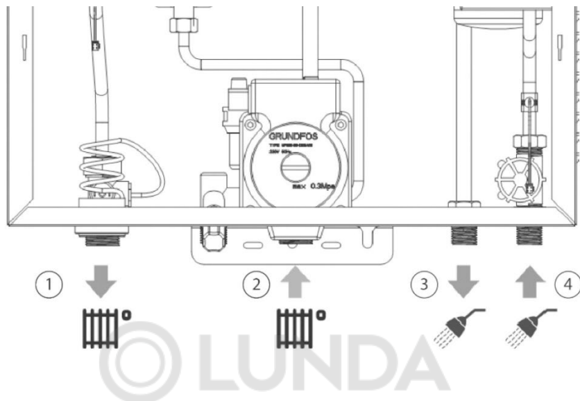
Рис. 6. Подключение к системам ГВС и отопления
