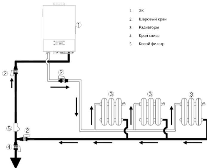
Рис. 7. Схема подключения «радиаторы + ЭК».
