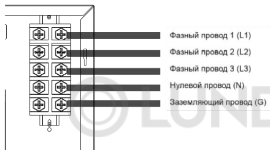
Рис.12. Подключение прибора
