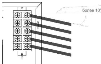
Рис. 13. Расположение сетевого кабеля
