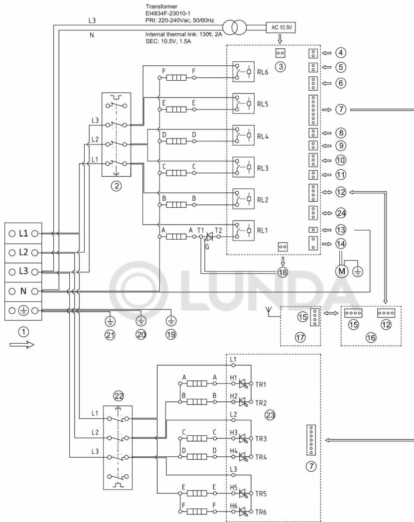
Рис.14. Электрическая схема
