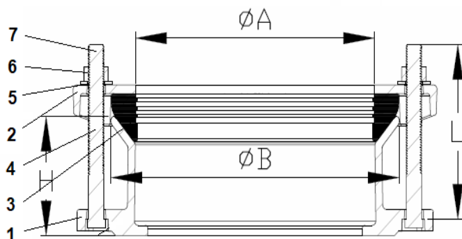
Рис.3. Муфта/адаптер ПФРК
