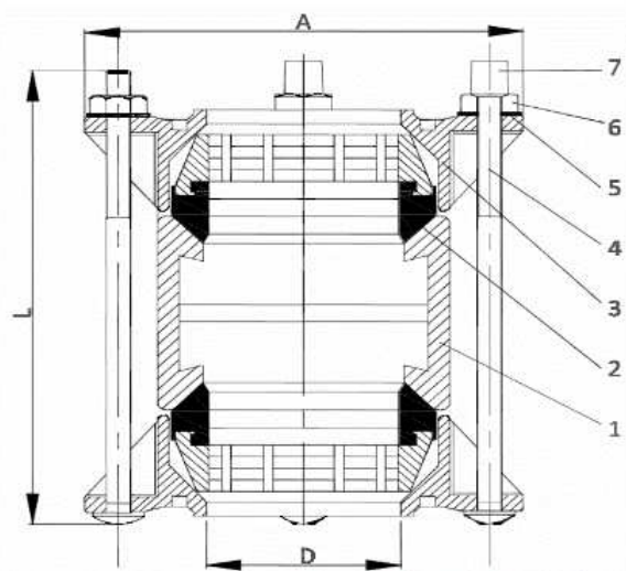
Рис.2. Муфта ДРК-Е
