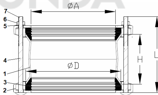
Рис.1. Муфта ДРК
