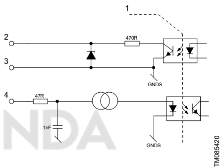
Схема аналогового интерфейса
