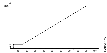
Профиль С входного ШИМ-сигнала (солнечные системы)
