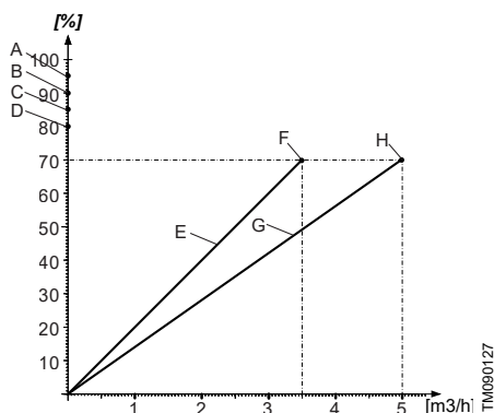
ШИМ-сигнал обратной связи — объемный расход
