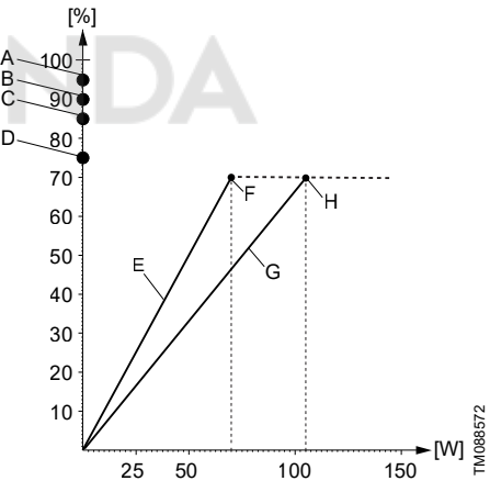
ШИМ-сигнал обратной связи — потребляемая мощность
