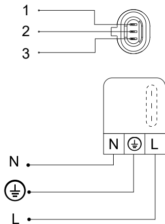
Штекерный разъем кабеля питания и сигнального кабеля
