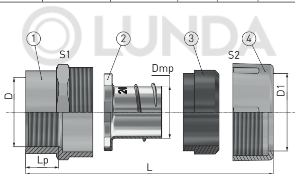
Рис. 3 – Резьбовой крепежный элемент с внутренней резьбой РКв: 1 – корпус; 2 – оконцеватель; 3 – уплотнитель; 4 – накидная гайка
