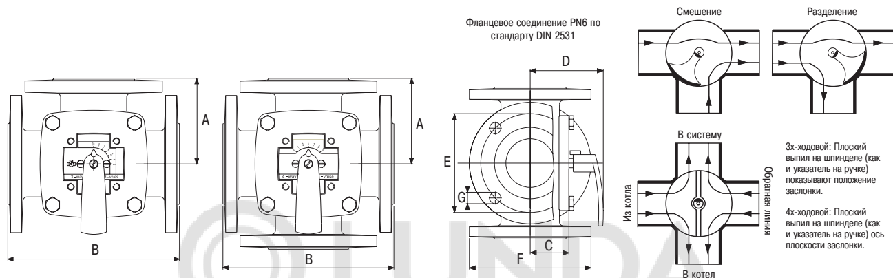
Размеры, 3х-ходовые клапаны
