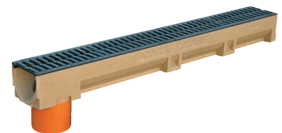
Канал ACO Euroline 1 м с чугунной решеткой
