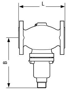
VFG2 (21), VFGS2 Д у 15–125
