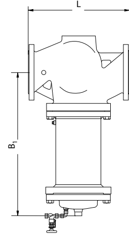
VFG2, VFGS2 Д у 150–250, с удлиненным штоком для T > 140 °C
