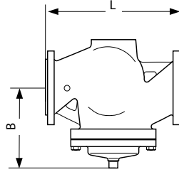
VFG2 (21), VFGS2 Д у 150–250
