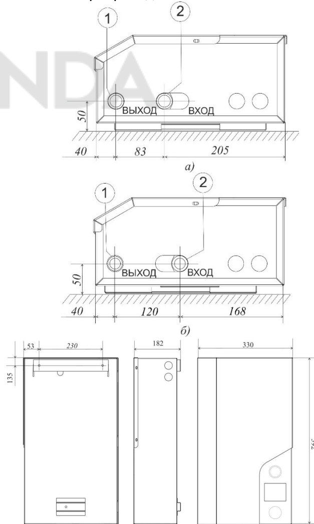
Рисунок 3 - Монтажные размеры электрокотла:
