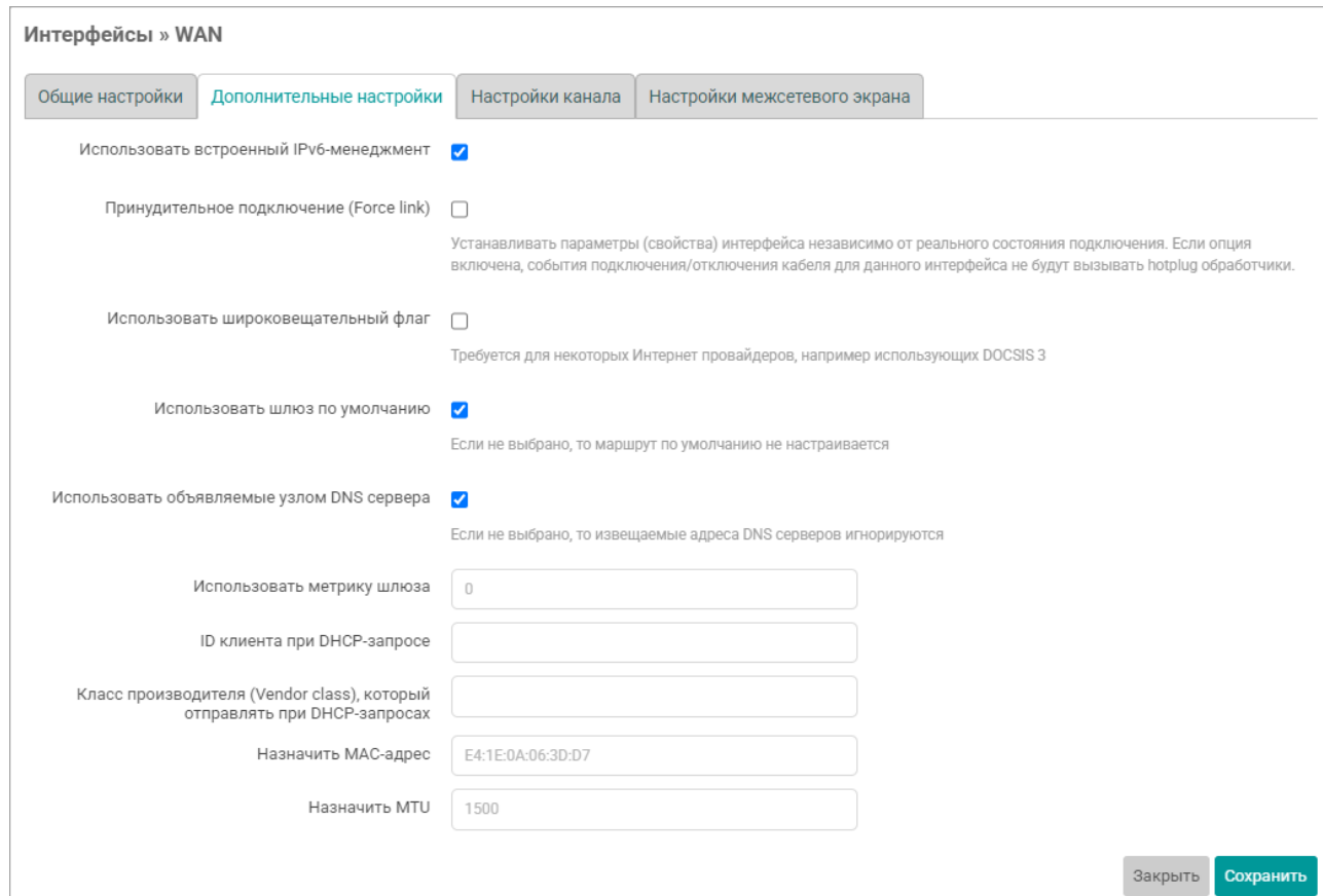
Рисунок 8.7 – Дополнительные настройки сетевого интерфейса для протокола DHCP-клиент
