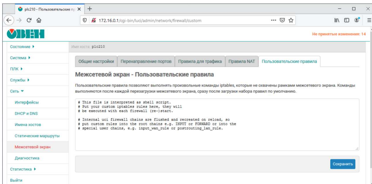
Рисунок 8.50 – Пользовательские правила межсетевого экрана
