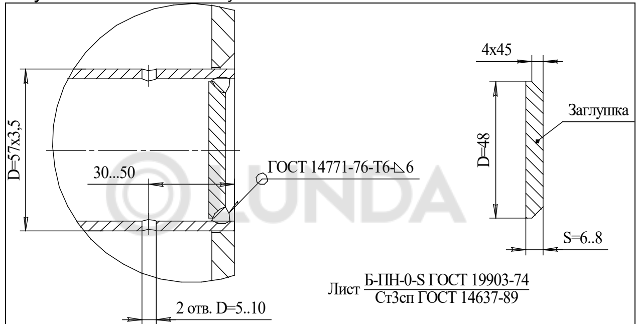
Рисунок 10. Установка заглушки.
