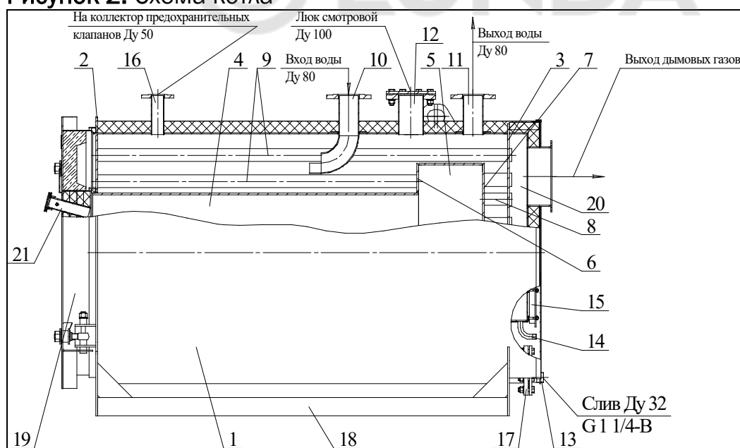
Рисунок 2. Схема котла
