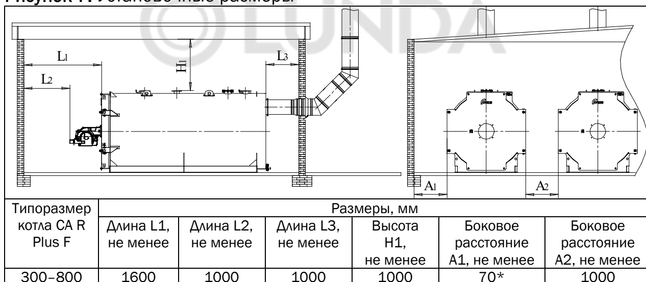
Рисунок 7. Установочные размеры
