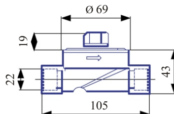
Рис.3 EAS для монтажа пайкой
