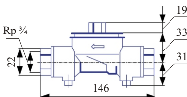
Рис.3 EAS с шаровыми кранами
