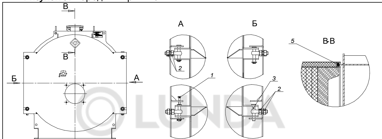
Рисунок 9. Передняя крышка.
