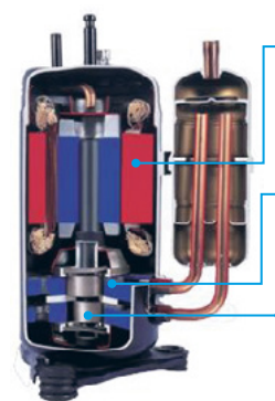
Двухроторный компрессор GMCC или Mitsubishi
