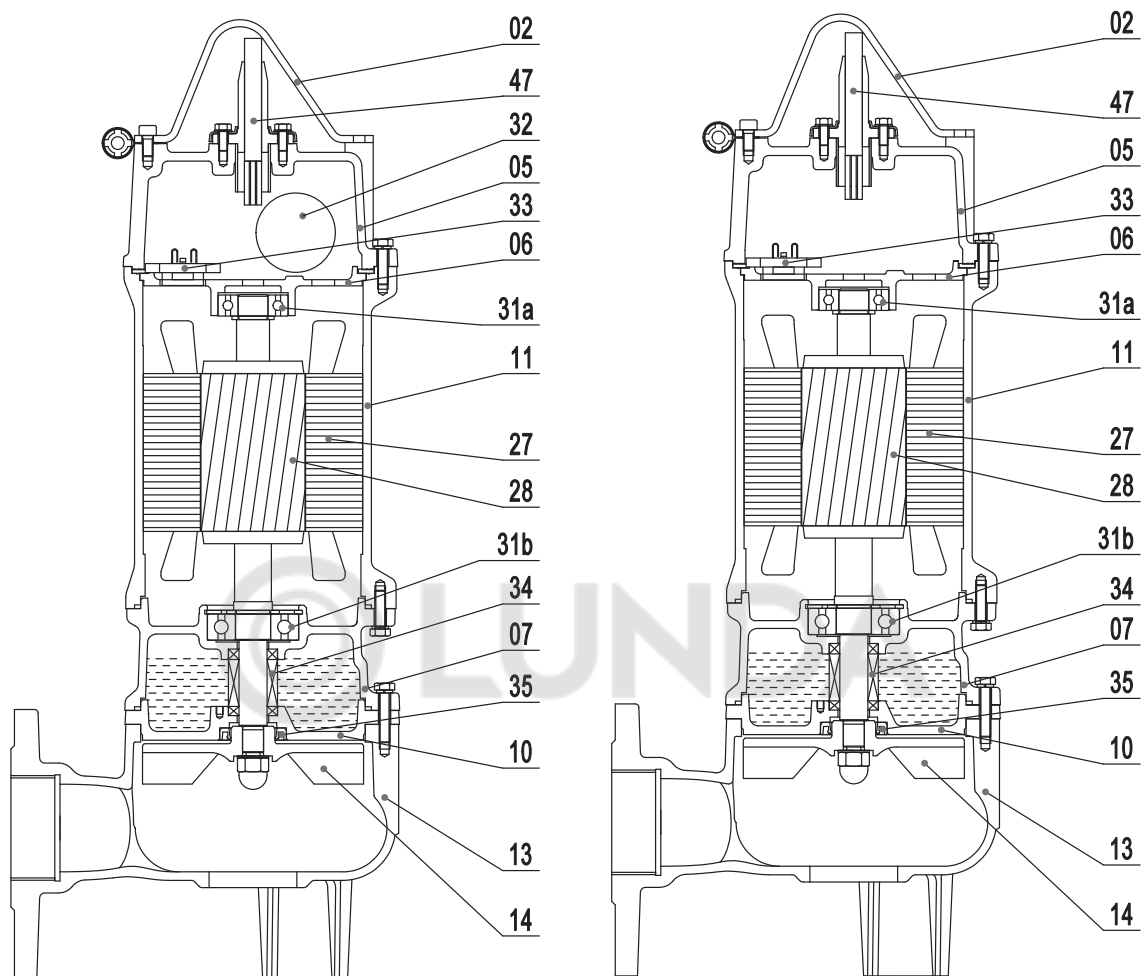
1-фазное исполнение
