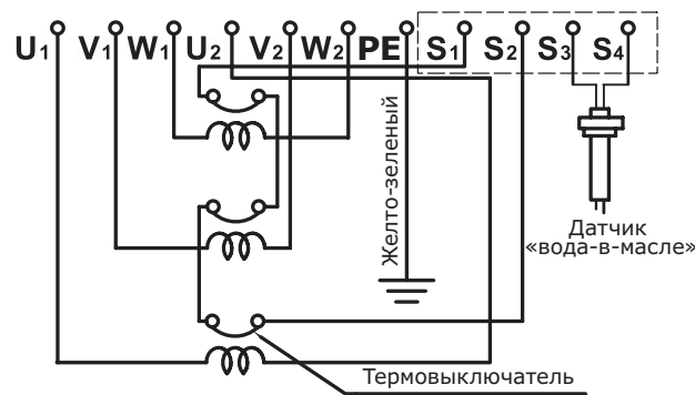
Пуск «звезда-треугольник», с биметаллическими термовыключателями и датчиком «вода-в-масле»
