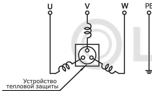
Прямой пуск, со встроенной тепловой защитой
