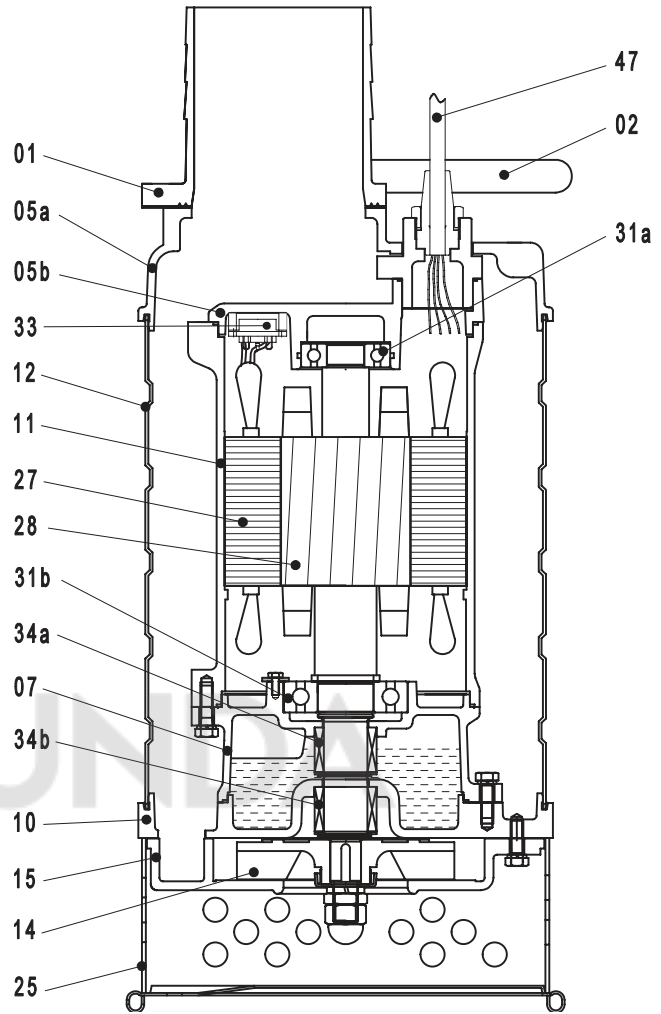
APV.09/12/20 3,7-11,0 кВт
