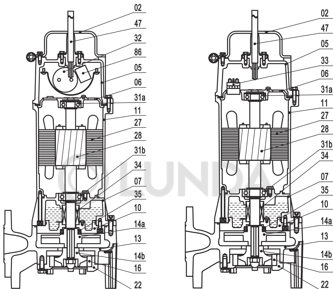
1-фазное исполнение
