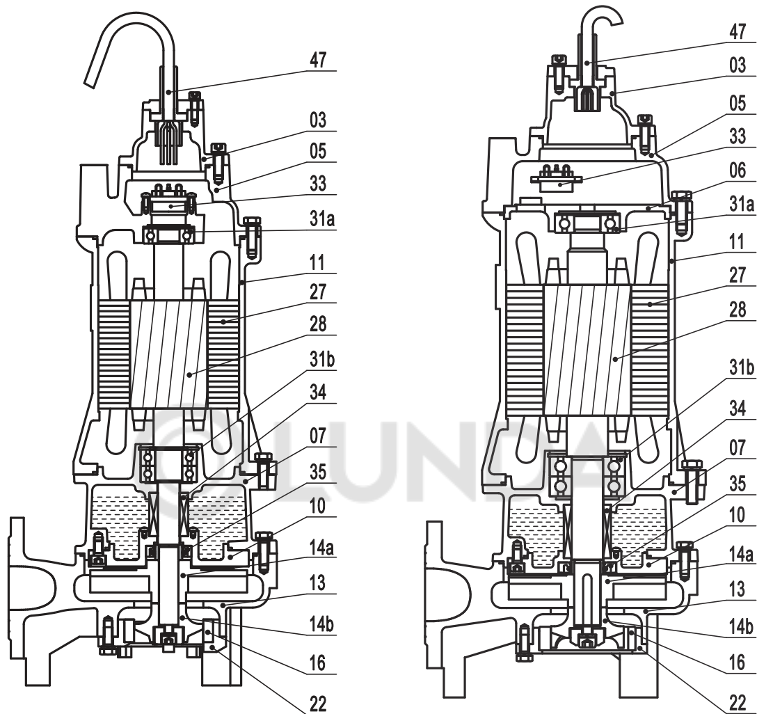
SG 1,5–2,2 кВт
