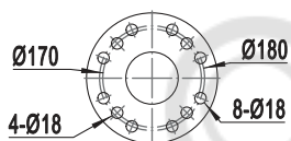
Фланец напорного патрубка насоса и переходника со стороны насоса DN100 PN6/ PN10
