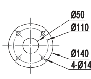
Размеры напорного патрубка насоса
