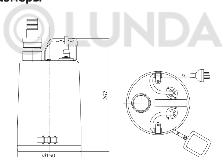
Рис. 5 Габаритные размеры APV.M.06.32.03.1 и APV.M.06.32.03.A1
