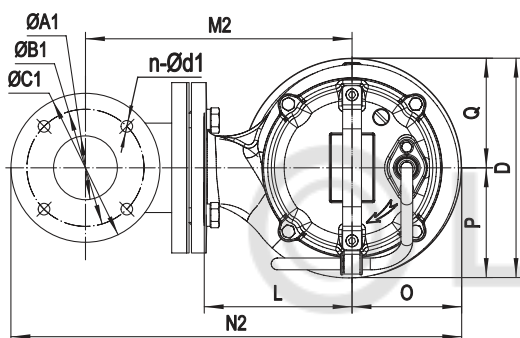
Размеры напорного патрубка насоса
