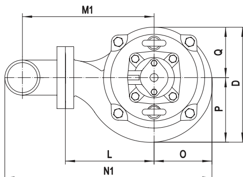
Фланцевое соединение с коленом
