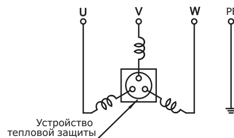
Схемы соединений с трехфазными двигателями
