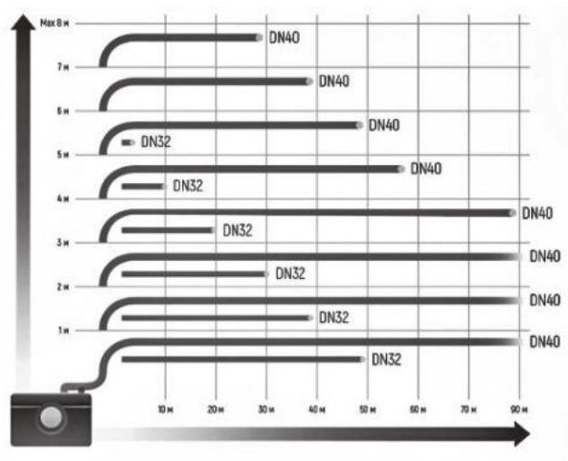
Рис. 31 Максимальная длина напорного трубопровода
