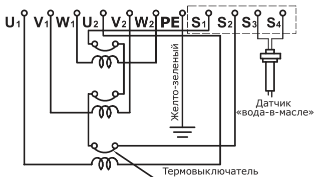
Схемы соединений с трехфазными двигателями
