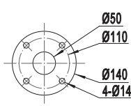
Размеры напорного патрубка насоса
