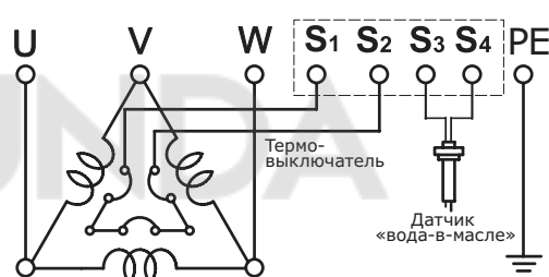
Схемы соединений с трехфазными двигателями
