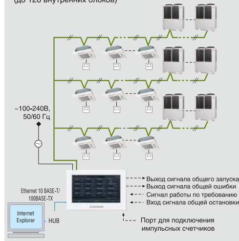
Схема системы (до 128 внутренних блоков)
