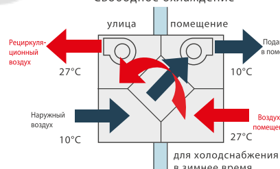
Принцип работы Свободное охлаждение
