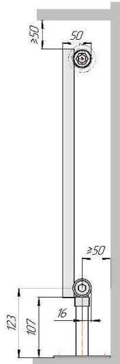
Гармония А 20-1 нп нв
