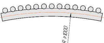
Гармония А 20-1 R наружн.
