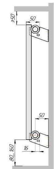
Гармония А 20-1 кронштейн Г-50
