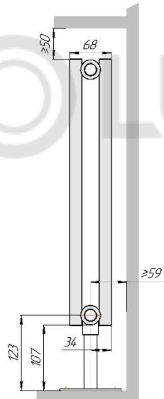
Гармония А 20-2 нв
