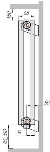
Гармония А 20-2 кронштейн Г-50
