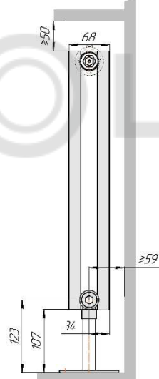
Гармония А 20-2 нп нв
