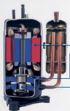
Двухроторный компрессор
