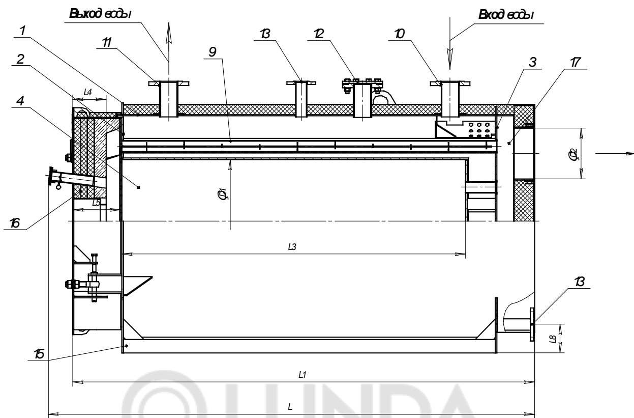
Рисунок 2. Схема котла (модуля)
