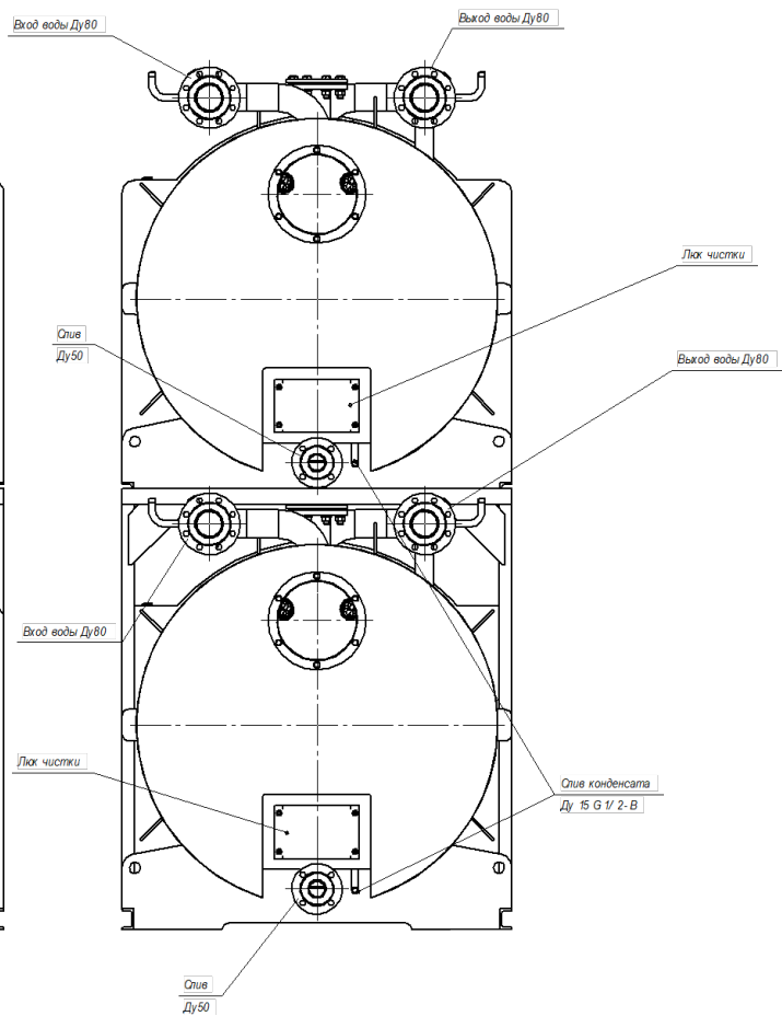
ВИД С ЗАДИ
