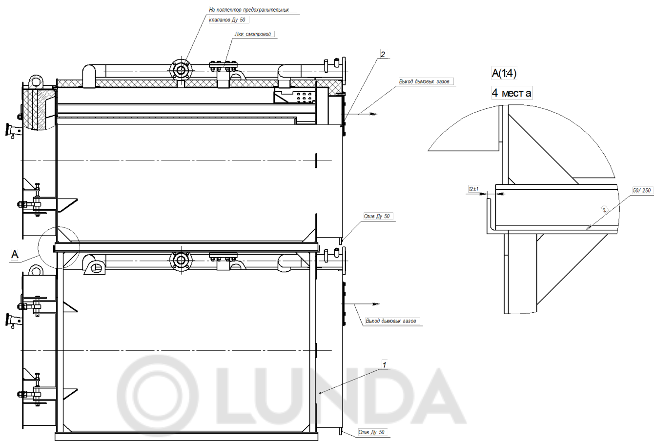
ВИД С ЗАДИ
