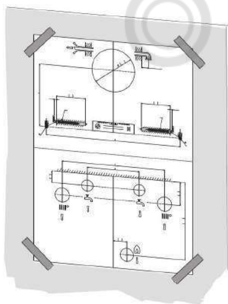
Рис. 31 Монтажный шаблон
