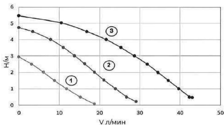
Рис.22 Характеристики насоса отопительного контура
