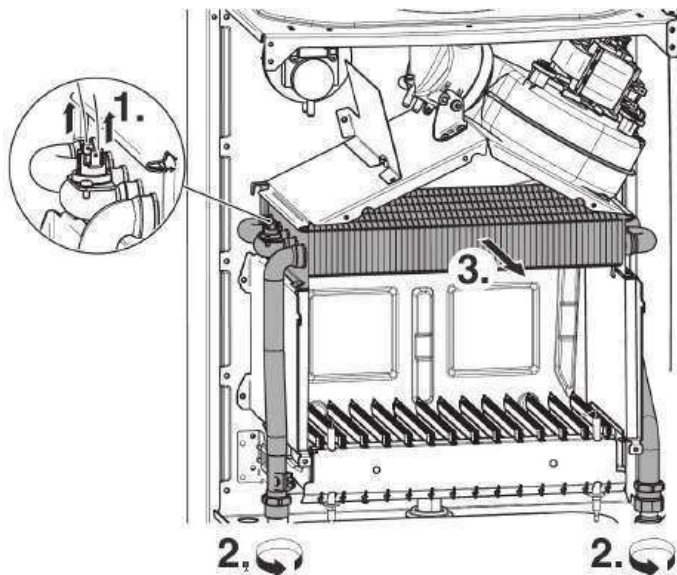
Рис.28 Чистка теплообменника
