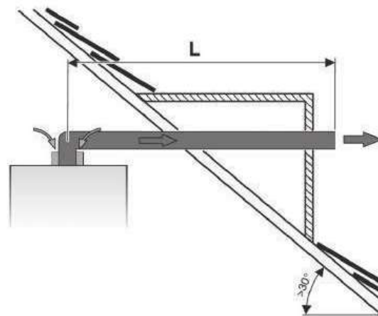
Рис. 3 Горизонтальный отвод дымовых газов B22
