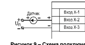
Рисунок 9 – Схема подключения пассивного датчика с токовым выходом 0...5 мА или 0(4)...20 мА
