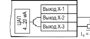
Рисунок 14 – Подключение к ВУ типа «И»
