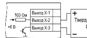
Рисунок 13 – Подключение нагрузки к ВУ типа «Т»
