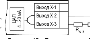
Рисунок 15 – Подключение к ВУ типа «И» с ограничивающим резистором
