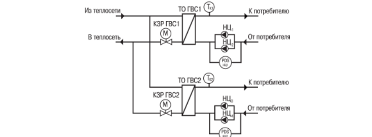
Рисунок 4 – Схема контура «Отопление + ГВС»
