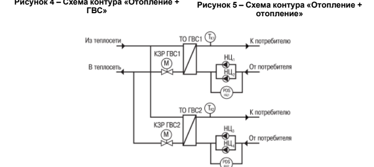
Рисунок 4 – Схема контура «Отопление + ГВС»
