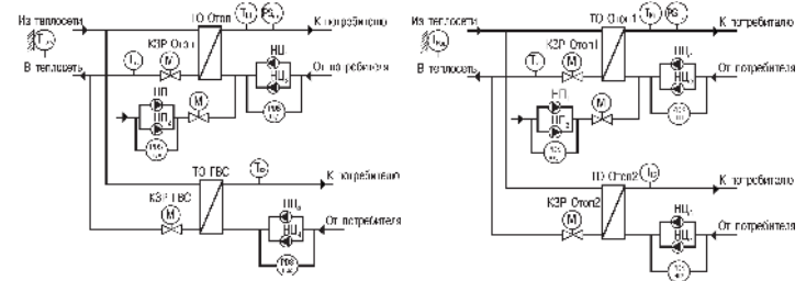
Рисунок 3 – Схема контура «ГВС»
