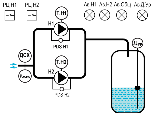
Рисунок 5 – Объект управления
