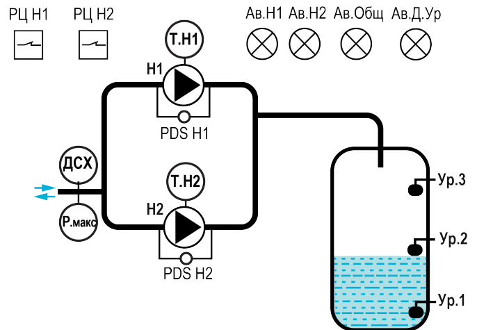
Рисунок 5 – Объект управления
