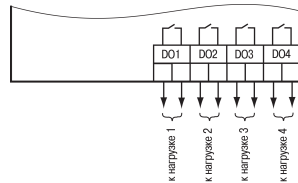
Рисунок 12 – Схема подключения нагрузки к ВЭ типа «Р»
