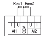
Рисунок 11 – Подключение резистивных датчиков
