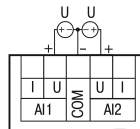
Рисунок 10 – Подключение датчиков с выходом в виде напряжения
