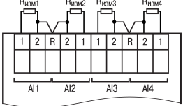
Рисунок 9 – Подключение резистивных датчиков
