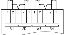
Рисунок 6 – Подключение ТС к AI PPM-x.3
