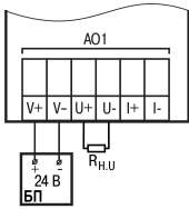
Рисунок 11 – Схема подключения к АО PPM-x.3 нагрузки типа У
