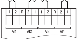
Рисунок 7 – Подключение ТП к AI PPM-x.3
