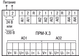
Рисунок 3 – Назначение контактов клеммника
