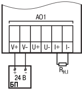
Рисунок 10 – Схема подключения к АО PPM-x.3 нагрузки типа И
