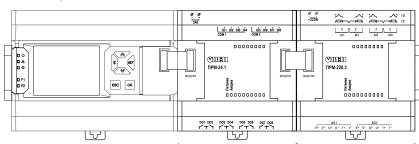
Рисунок 16 – Расположение модулей расширения на шине
