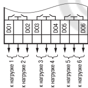
Рисунок 9 – Схема подключения ВЭ типа «Р»
