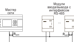
Рисунок 14 – Типовая схема подключения в режиме Master
