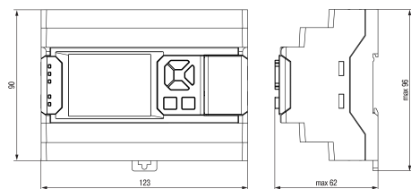
Рисунок 1 – Габаритные размеры прибора
