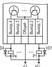
Рисунок 9 – Подключение нагрузки к ВЭ типа «К»
